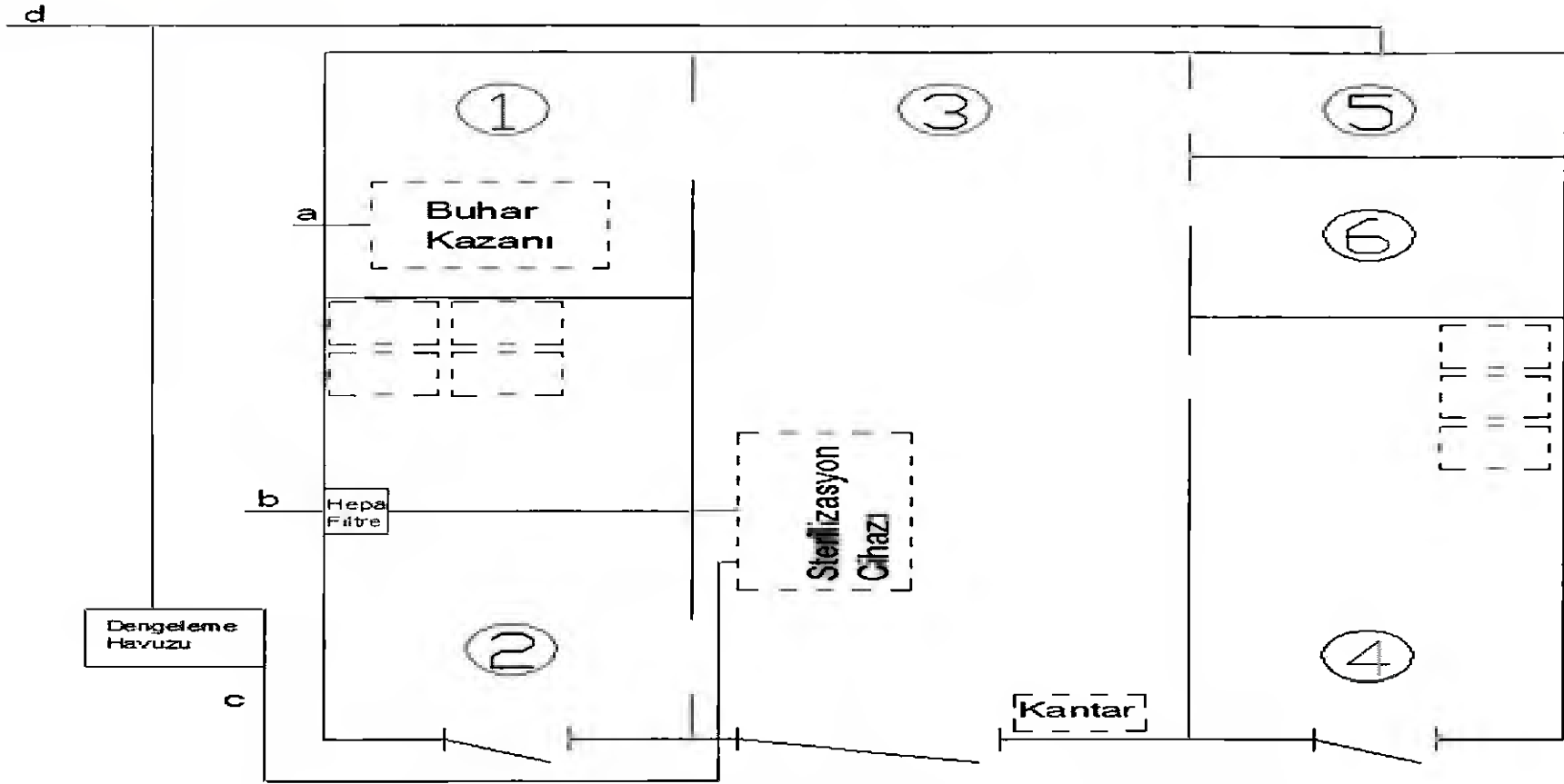
Şekil 1: Tıbbi Atık Sterilizasyon Ünitesi Vaziyet Planı
